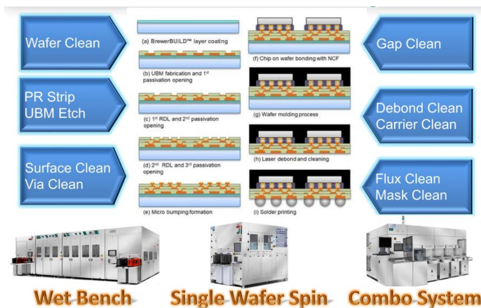
圖表一、弘塑產品以及應用於 CoW 製程站點
